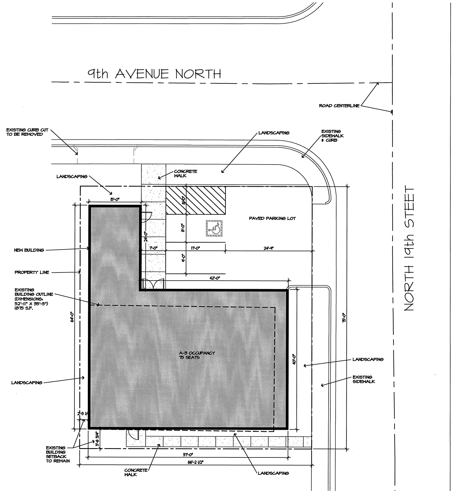
1 SITE PLAN 2640 S.F. A-1 Scale: 1/16" = 1'-0"
