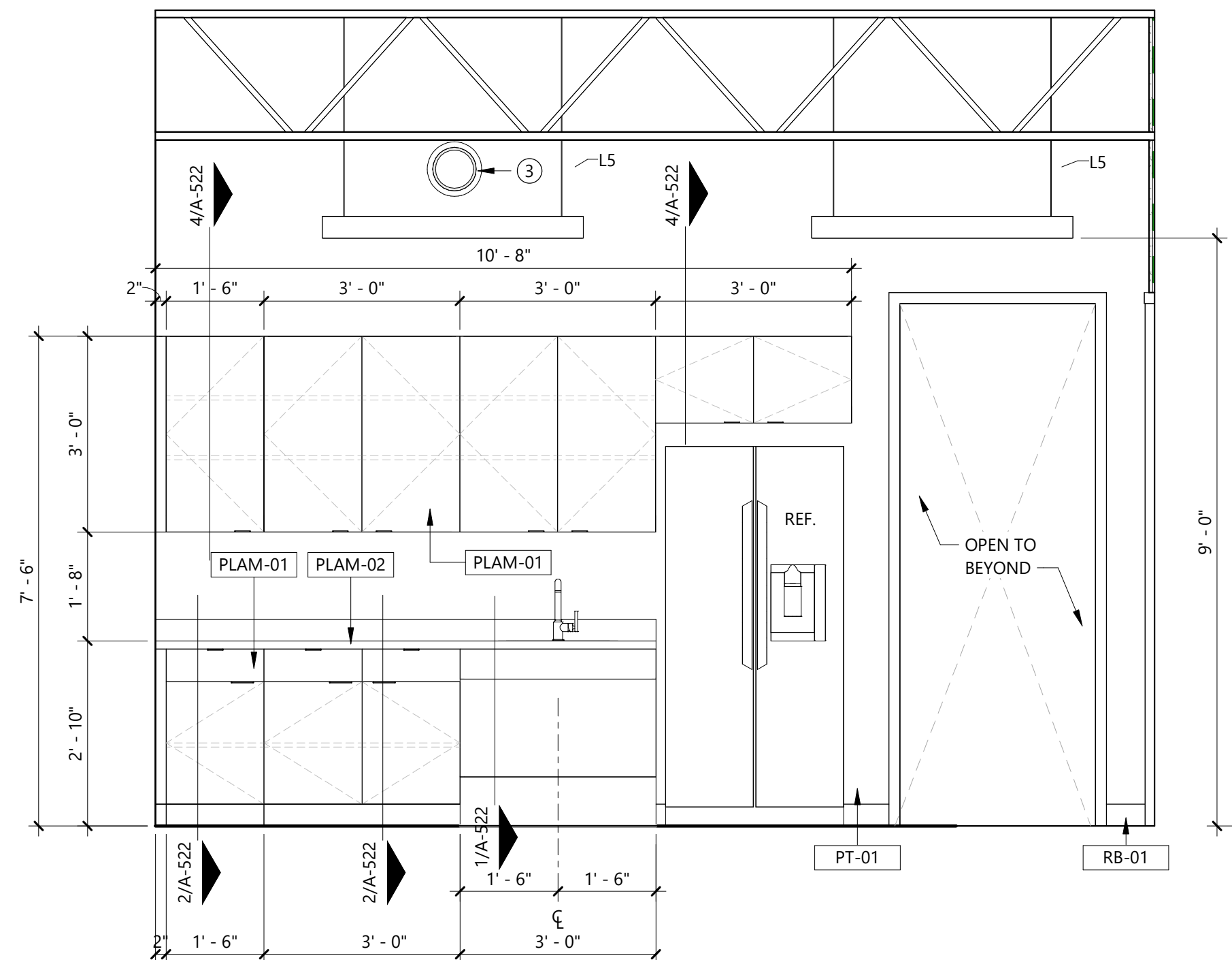
1 BREAKROOM SCALE: 1/2" = 1'-0"
