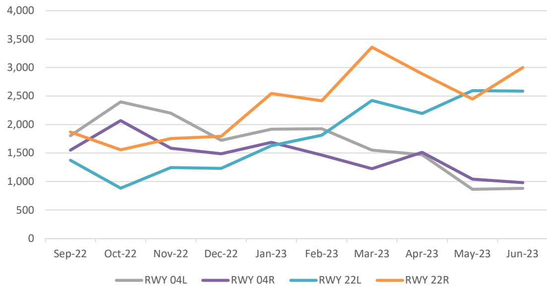
Landings per RWY
