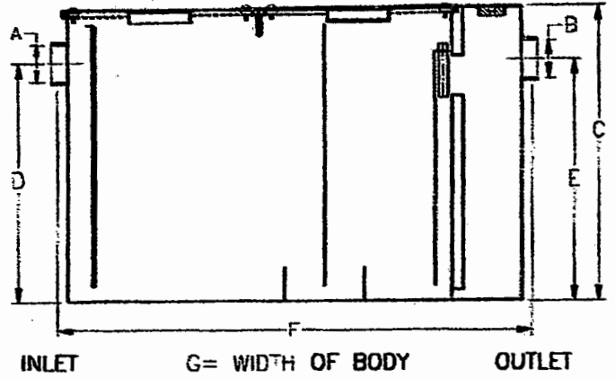
GT2700-75 & GT2700-100
