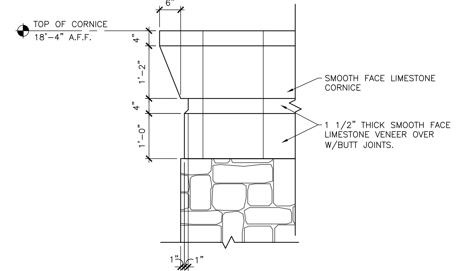
4 CORNICE DETAIL SCALE: 3/4"=1'-0"
