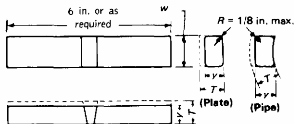
Root-bend specimen
