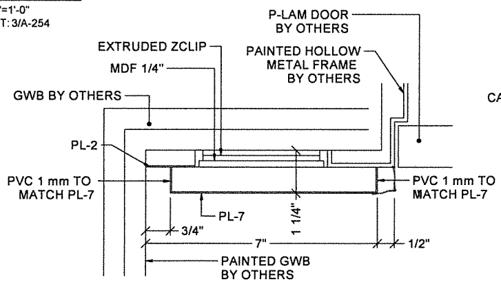
5 SECTION TYP SK-10 SCALE: 3"=1'-0" REF ARCHIT: A11/A-559
