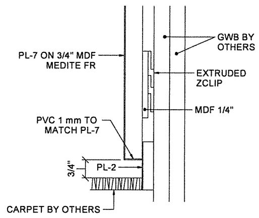
4 SECTION TYP SK-10 SCALE: 3"=1'-0" REF ARCHIT: A15/A-559
