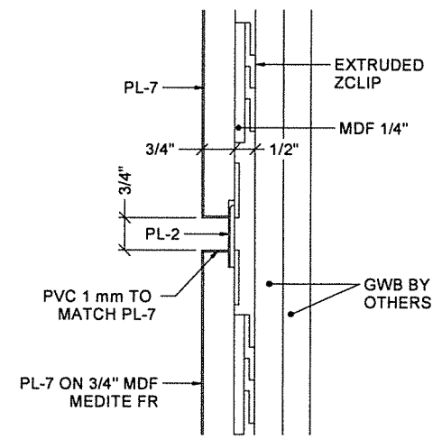
3 SECTION TYP SK-10 SCALE: 3"=1'-0" REF ARCHIT: A12/A-559
