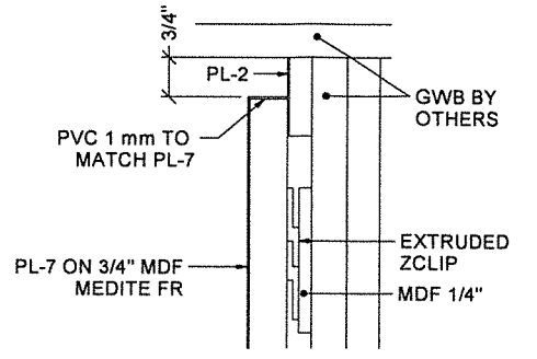
2 SECTION TYP SK-10 SCALE: 3"=1'-0" REF ARCHIT: A16/A-559
