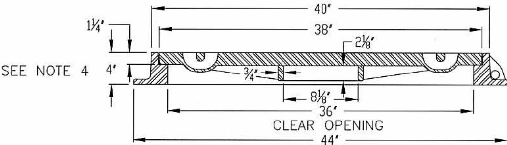
SECTION A-A
