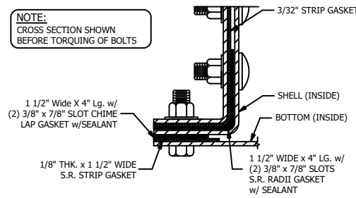
GASKET SECTION B-1 N.T.S.
