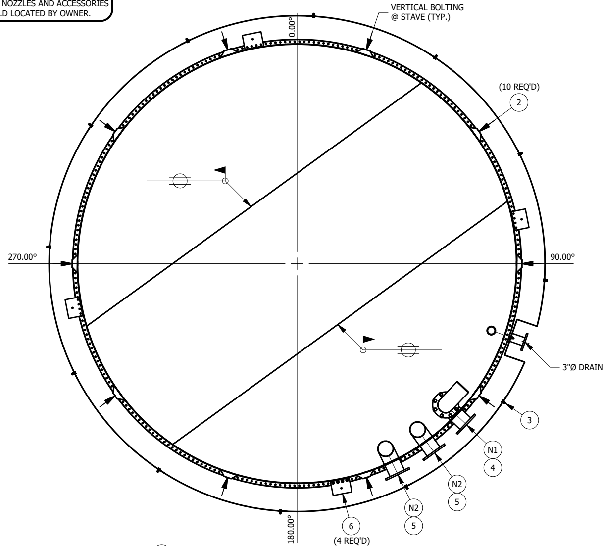
PLAN ORIENTATION N.T.S.
