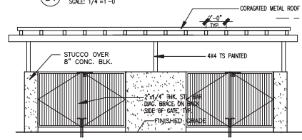
B FRONT ELEV. SCALE: 1/4" = 1'-0"
