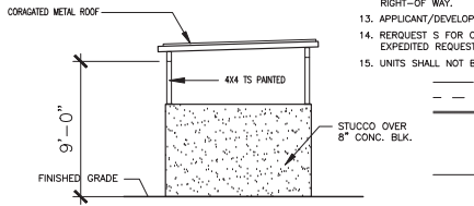
B1 SIDE ELEV. SCALE: 1/4" = 1'-0"
