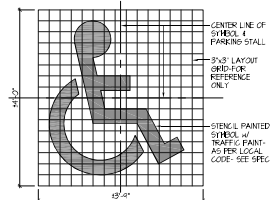
2 TYP. ADA DETAIL
