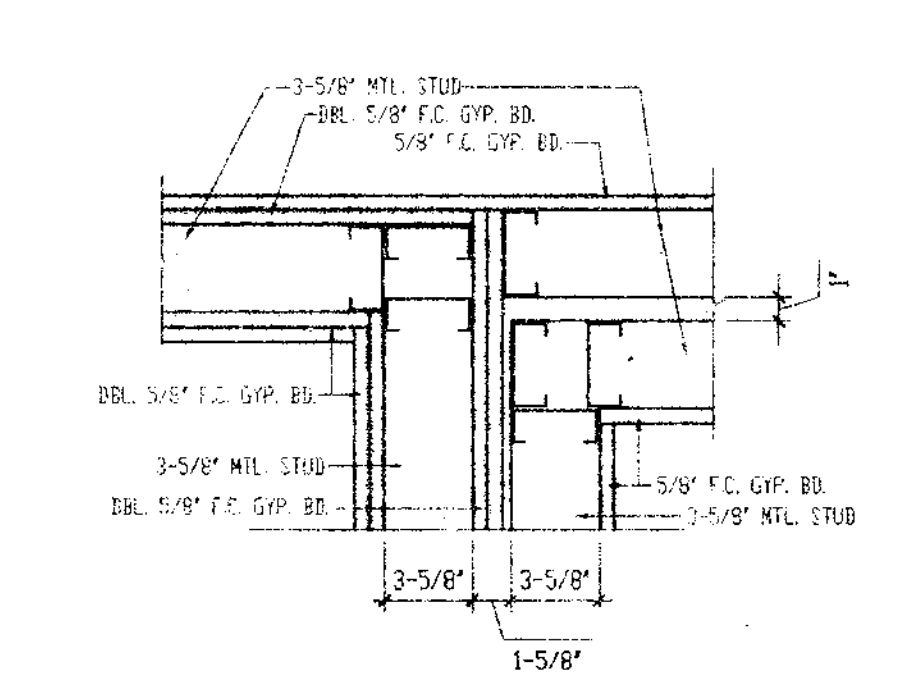
4 2 HR. WALL DETAIL SCALE: 3" = 1'-0"
