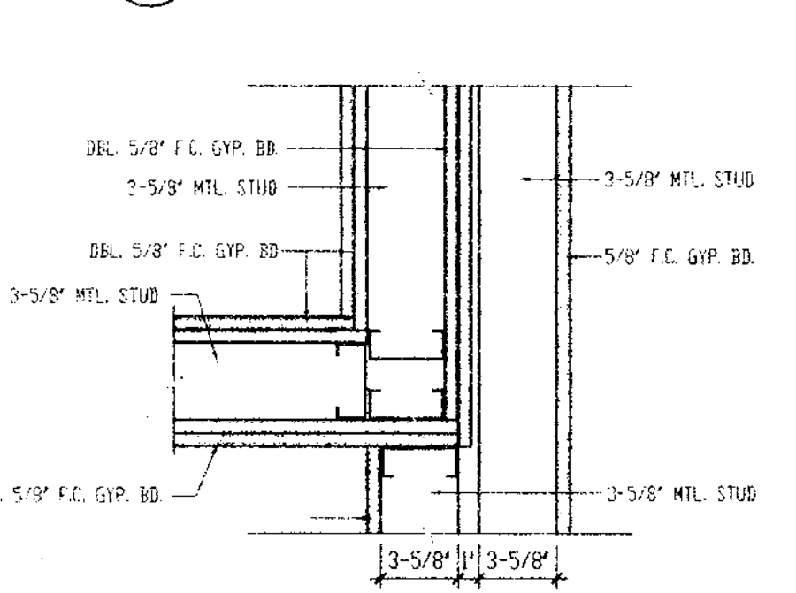
2 2 HR. WALL DETAIL SCALE: 3" = 1'-0"
