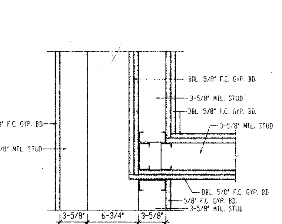
2 2 HR. WALL DETAIL SCALE: 3" = 1'-0"
