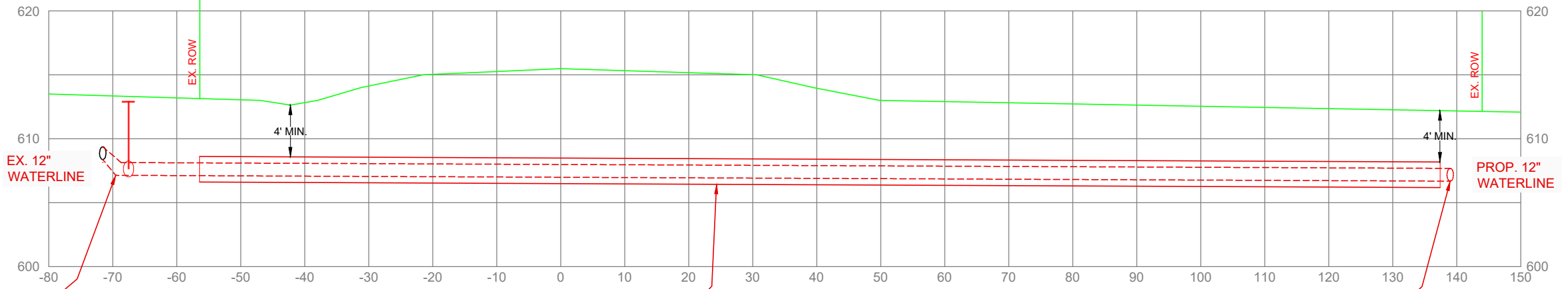
FM 973 STA. 519+54
