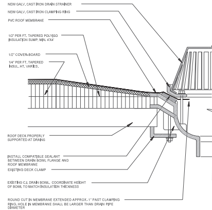
5 SUMPED ROOF DRAIN SCALE: N.T.S.
