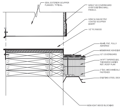
5 THRU WALL ROOF OVERFLOW SCUPPER SCALE: N.T.S.
