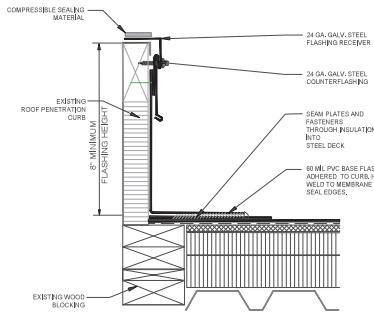
1 EXISTING EQUIPMENT CURB FLASING SCALE: N.T.S.
