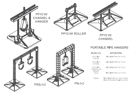
3 ROOFTOP PIPE SUPPORTS SCALE: N.T.S.
