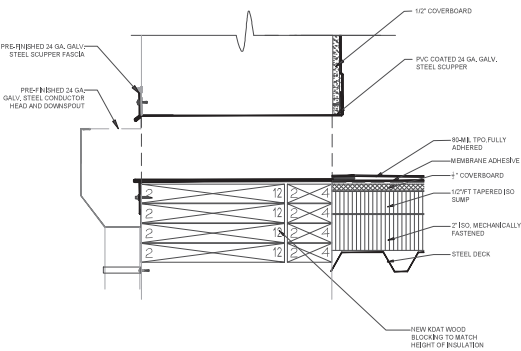
4 THRU WALL ROOF SCUPPER SCALE: N.T.S.
