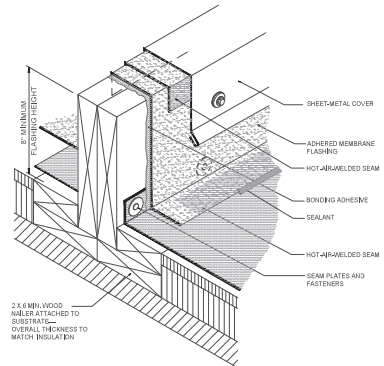
6 THRU WALL ROOF OVERFLOW SCUPPER SCALE: N.T.S.
