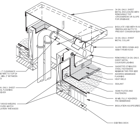
4 PIPE/CONDUIT PENETRATION CURB SCALE: N.T.S.
