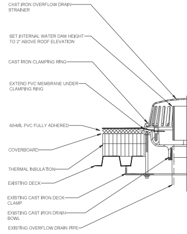
6 OVERFLOW ROOF DRAIN SCALE: N.T.S.
