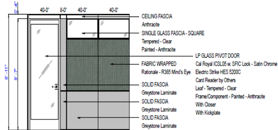
Elevation B
