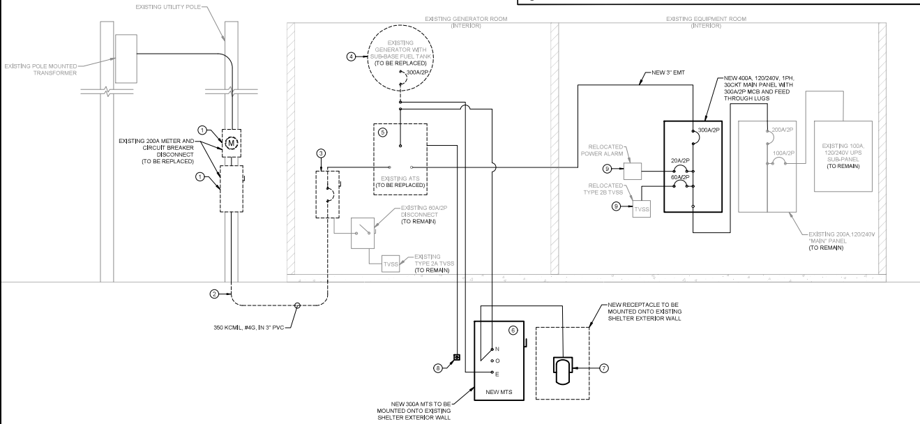
1 ELECTRICAL ONE-LINE DIAGRAM SCALE: N.T.S.
