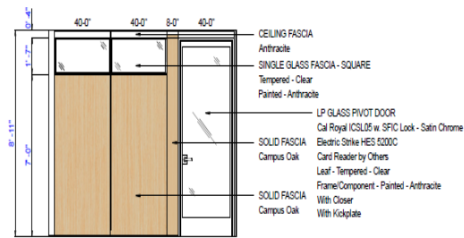
Elevation A
