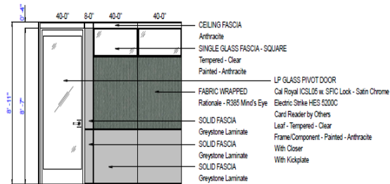
Elevation B
